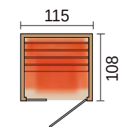
Außenmaße B 115 x T 108 x H 206 cm
